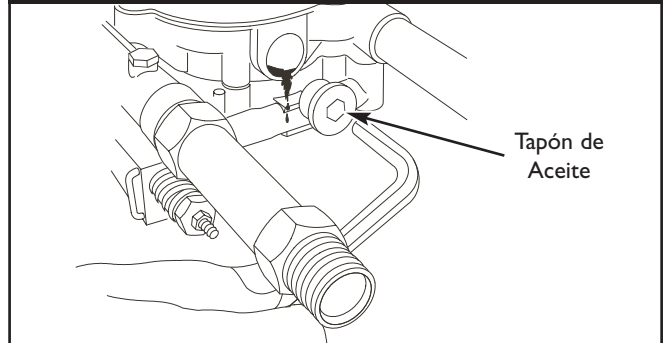
Figura 45 - Cambio del Aceite de la Bomba
