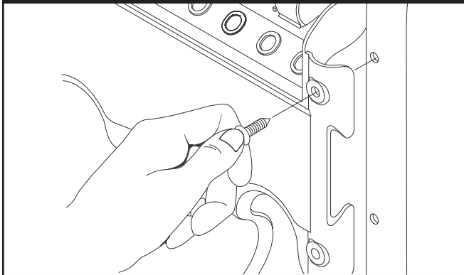
Figura 26 - Conecte Bandeja Accesoría
